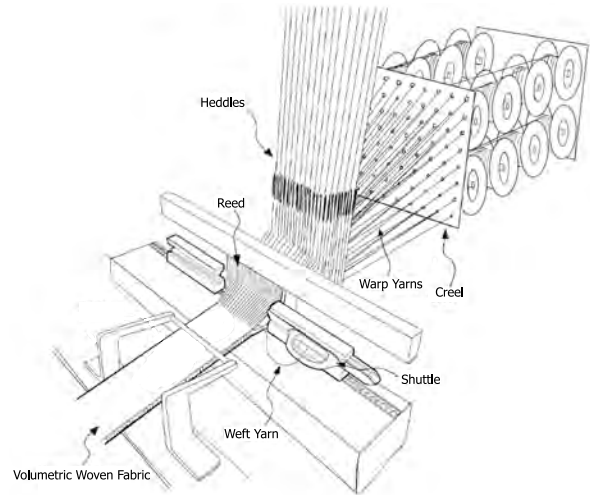
Fig. 3. Jacquard Loom
